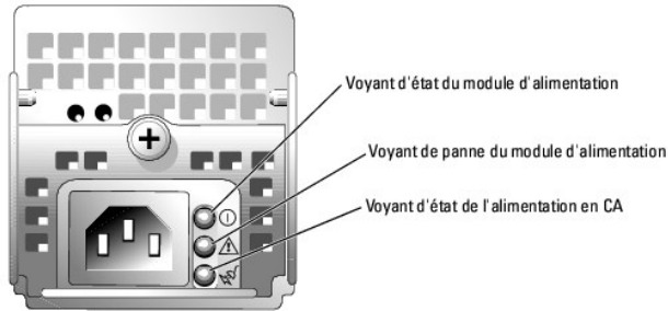
Figure 1-4. Voyants des modules d'alimentation redondants
