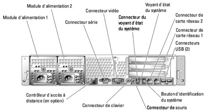
Figure 1-3. Éléments et voyants du panneau arrière
