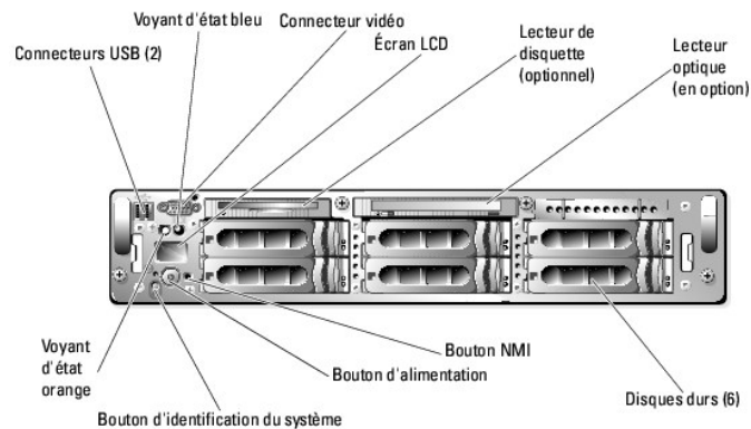
Figure 1-1. Éléments et voyants du panneau avant
